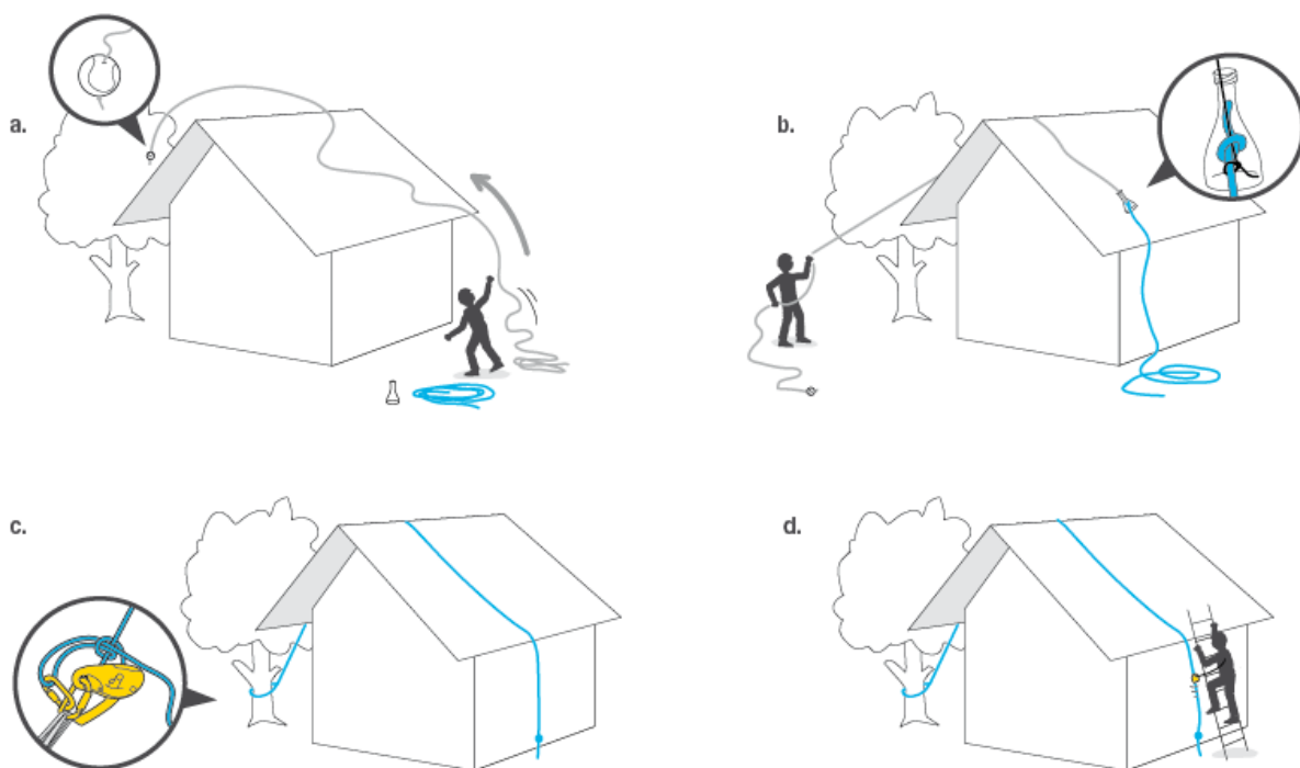
8. Predisposizione accesso su copertura in assenza di presidi di dotazione dell'opera
